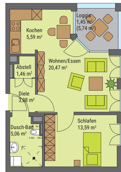
Beispiel für eine 1-Personen-Wohnung, 50,71 m 2 im 2. Obergeschoss
